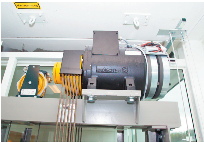
Växellös hissmaskin placerad i schakttopp
