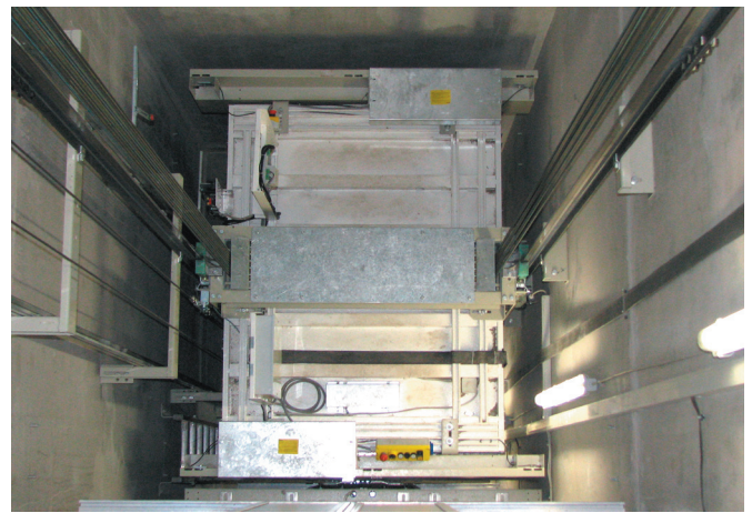
Hisskorg i schakt med gejder på två sidor i 2:1 utförande
